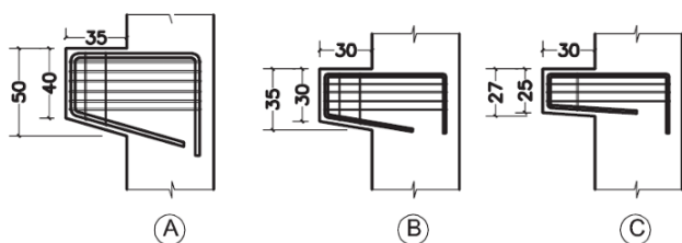
Figura 2.24: Mensulas.
