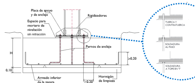
Figura 2.18: Nudo Cimentación.
